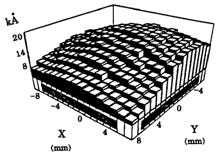
Figure 4: Distribution en épaisseur d'un film sur substrat Silicium
