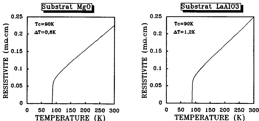
Figures 5 et 6: Caractéristiques électriques de films supraconducteurs
