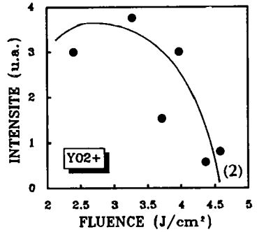
Figures 1 et 2: Evolution de l'intensité avec la fluence
